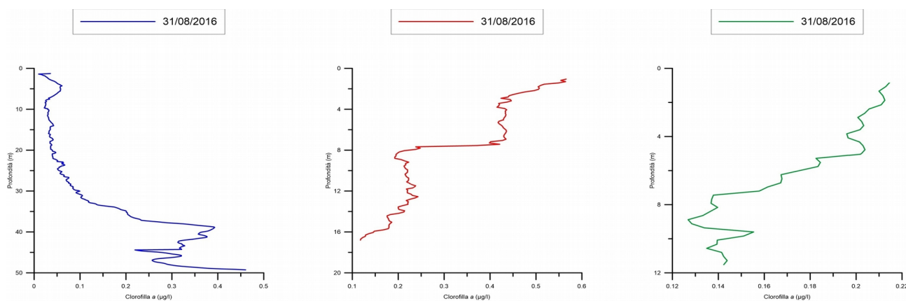
Fig. 10 Andamento della Clorofilla a nelle Stazioni ST03PT, ST02PT, ST01PT durante la campagna FPOA_18
