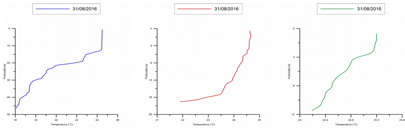
Fig. 4 Andamento della Temperatura nelle Stazioni ST03PT, ST02PT, ST01PT durante la campagna FPOA_18
