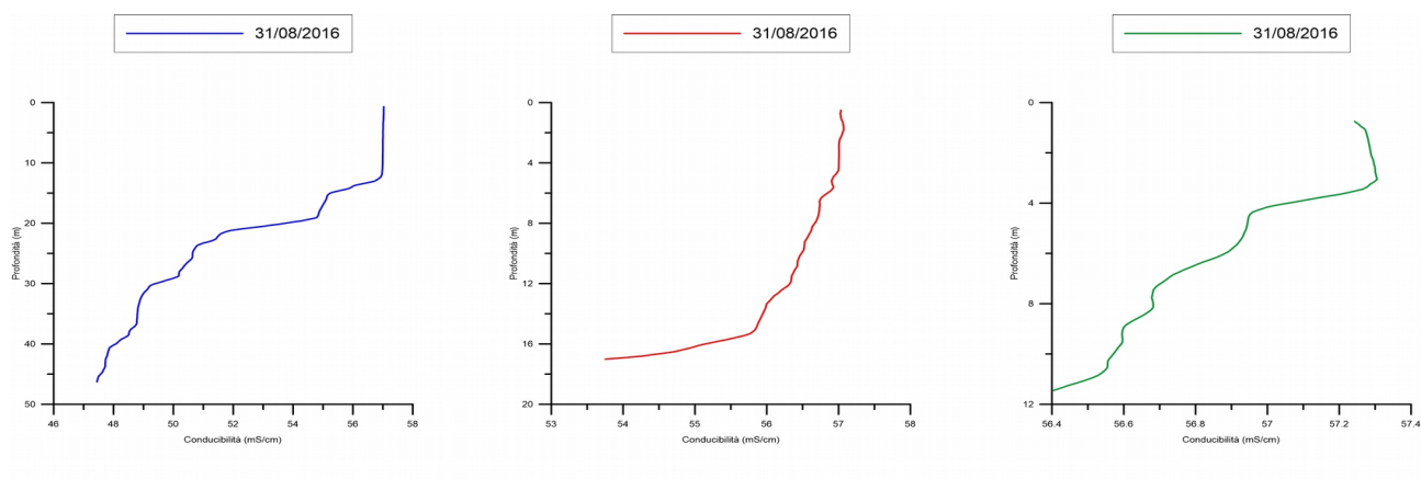
Fig. 5 Andamento della Conducibilità nelle Stazioni ST03PT, ST02PT, ST01PT durante la campagna FPOA_18
