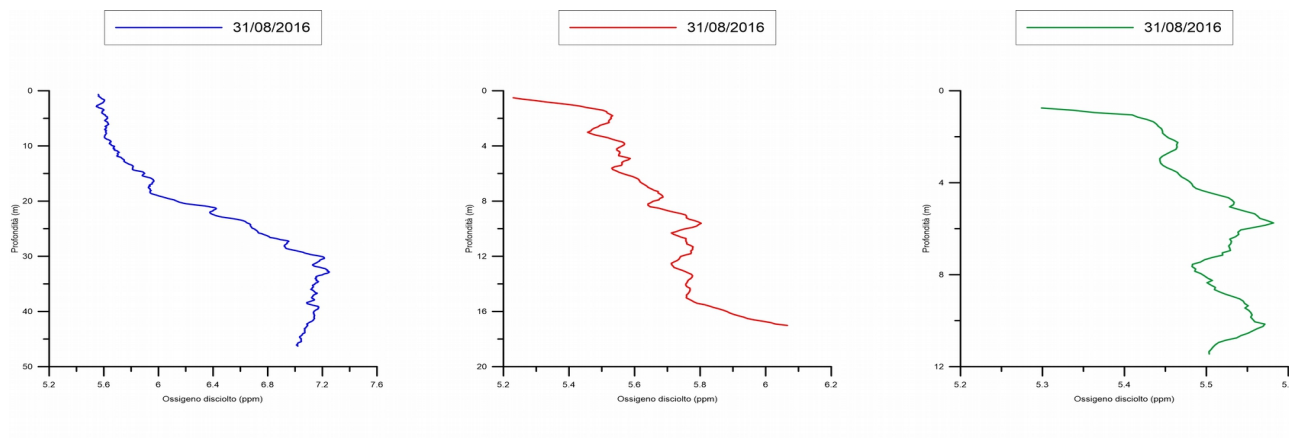
Fig. 8 Andamento dell'Ossigeno disciolto nelle Stazioni ST03PT, ST02PT, ST01PT durante la campagna FPOA_18
