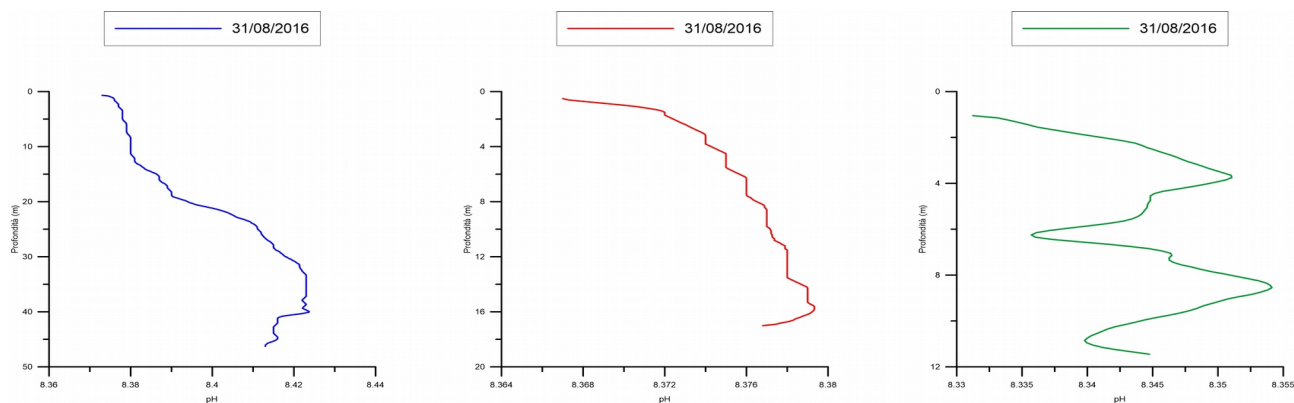
Fig. 9 Andamento del pH nelle Stazioni ST03PT, ST02PT, ST01PT durante la campagna FPOA_18
