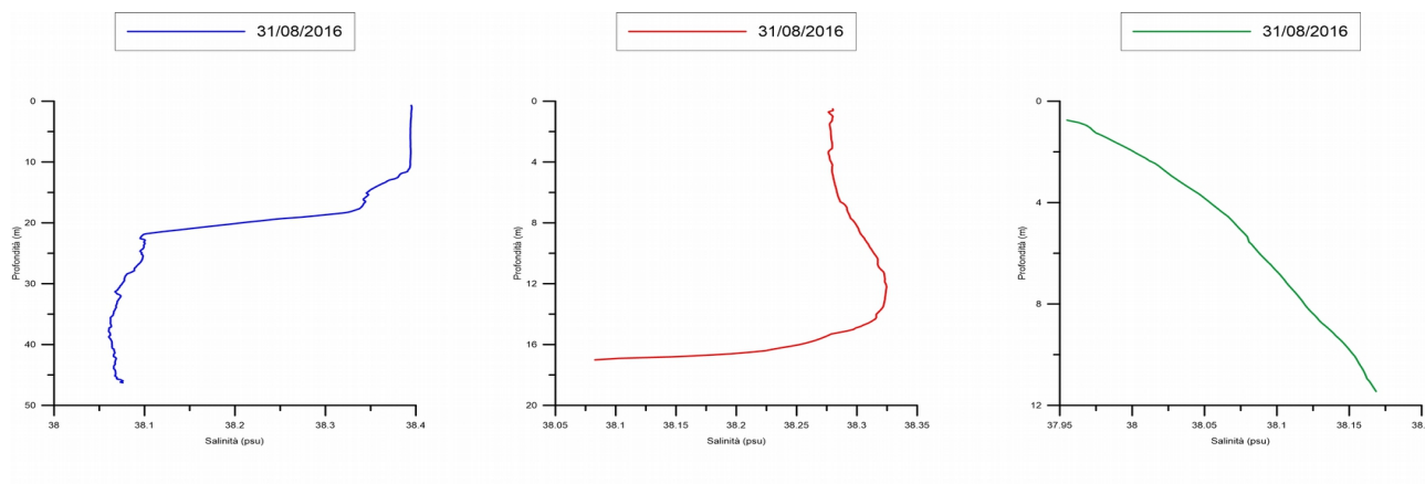
Fig. 6 Andamento della Salinità nelle Stazioni ST03PT, ST02PT, ST01PT durante la campagna FPOA_18
